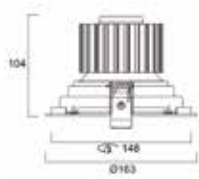
Expospot 90mm Unitario Redondo Cardán
