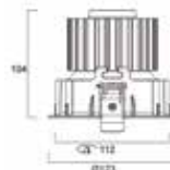
Expospot 90mm Fijo
