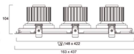
Expospot 90mm triple Cuadrado cardán
