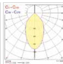
Expospot 90 Fixe HO RA80 4,000K WB Blanc
